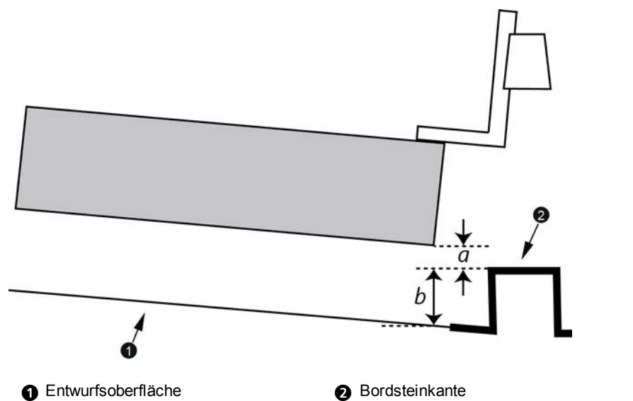
Abbildung 4.2 Messungen für die Höheneinstellung eines Sonic Tracers über einer Bordsteinkante
