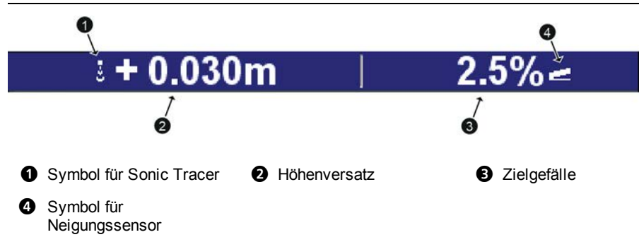
Abbildung 2.3 Beispiel für einen Bereich mit Führungseinstellungen für ein mit Sonic Tracer geführtes System „Heben + Querneigung“
